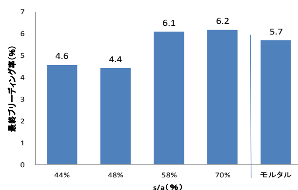
図-3 最終ブリーディング率
