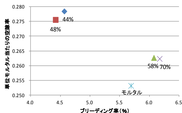
図-5 ブリーディングと単位モルタル当たりの空隙率の関係
