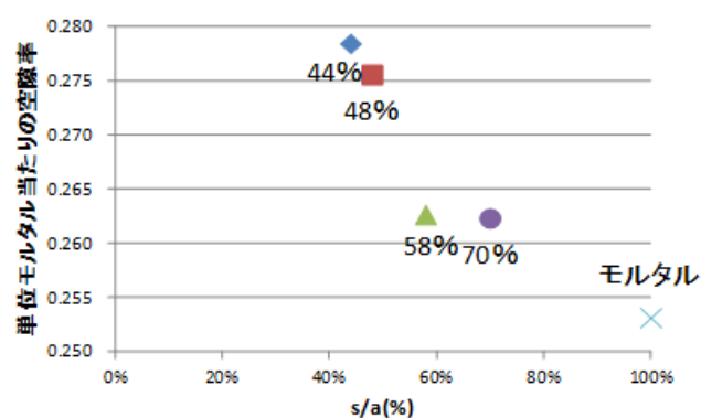
図-4 s/a と単位モルタル当たりの空隙率の関係
