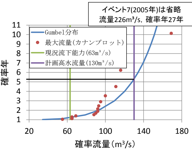
図-7 改修完了後の治水安全度
