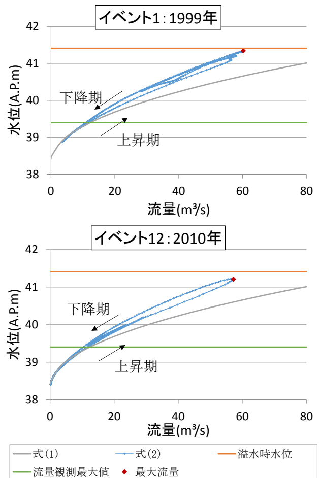
図-4 水位流量曲線の例
