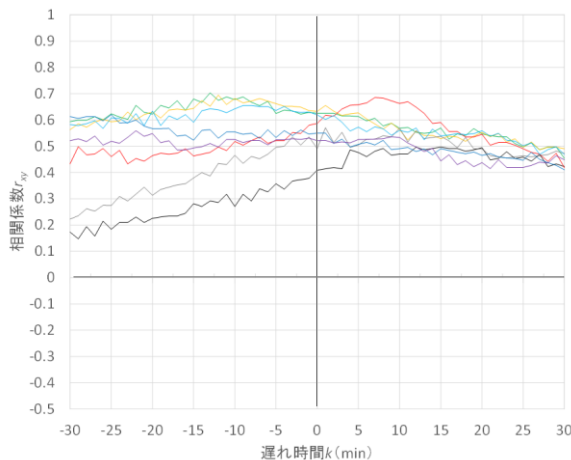
図-6 No.11の相互相関関数 r_{xy}
