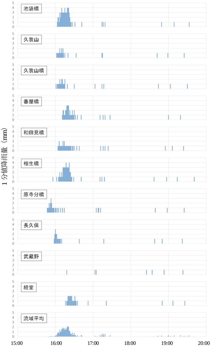
図-3 豪雨イベント No.1 のハイトグラフ
