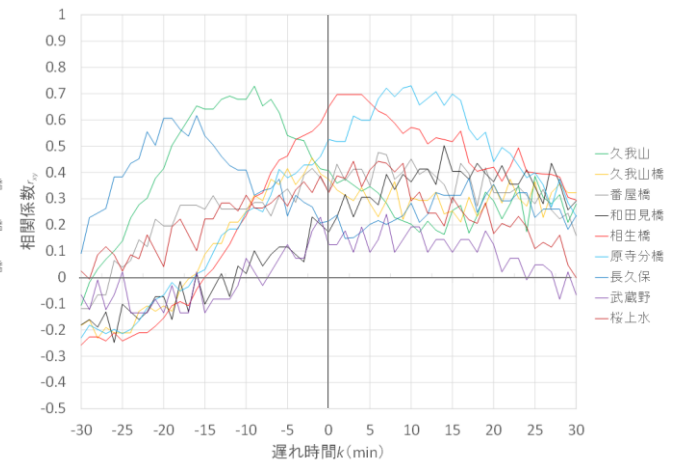
図-5 No.1の相互相関関数 r_{xy}
