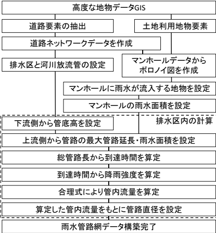
図-2 データ構築のフローチャート
