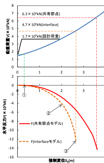
図.9 複合主塔終局強度特性
