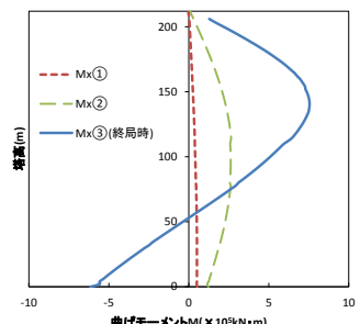
図.11 曲げモーメント分布
