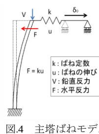
図.4 主塔ばねモデル
