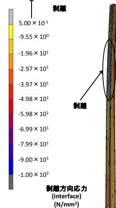
図.10 終局時剥離分布図
