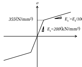
図.6 構成則 (SM490Y)
