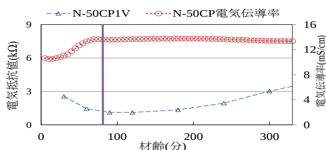
図4 セメントペーストの電気抵抗値と伝導率
