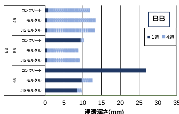
図-3 塩水浸漬試験結果
