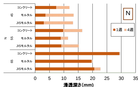
図-2 非定常電気泳動試験結果
