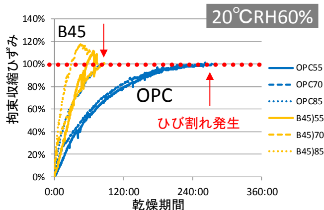
図-3 拘束収縮ひずみと乾燥期間の関係
