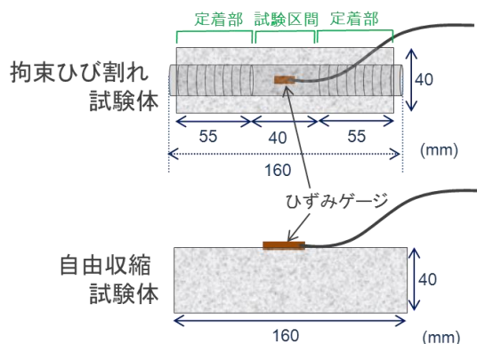
図-1 試験体概要
