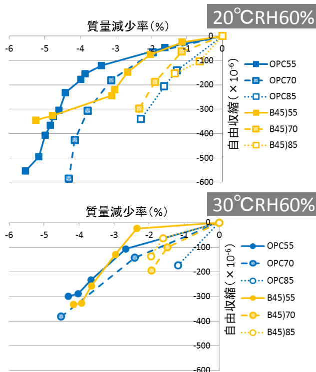
図-4 質量減少率と自由収縮 (上:20℃, 下:30℃)
