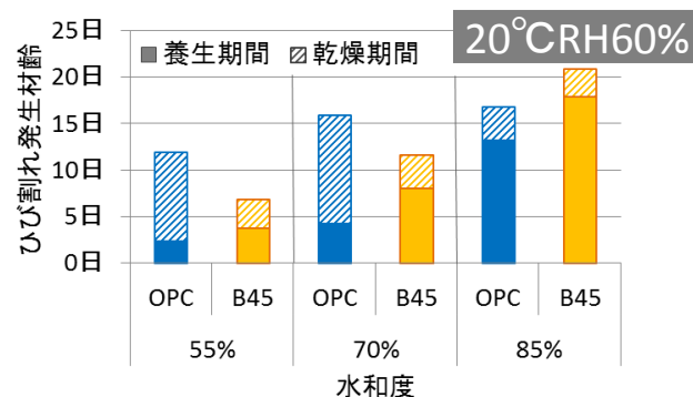
図-2 水和度とひび割れ発生材齢の関係
