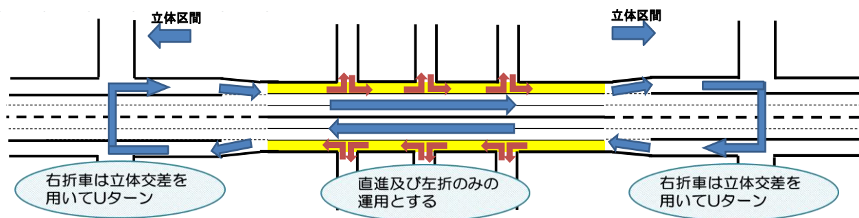
図-4 緩速車線を適用した交通運用策
