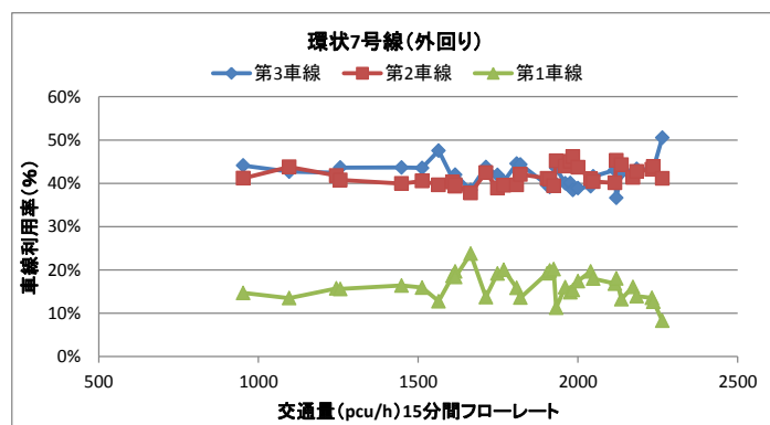
図-5 各車線の車線利用率の推移
