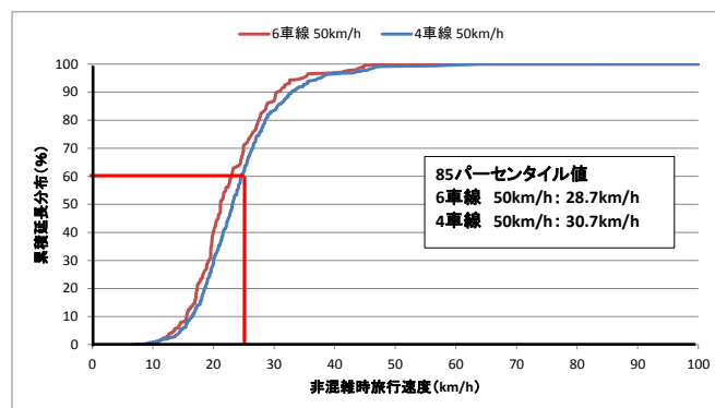
図-1 多車線道路のサービス状況
