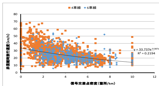
図-2 信号交差点密度と旅行速度の関係
