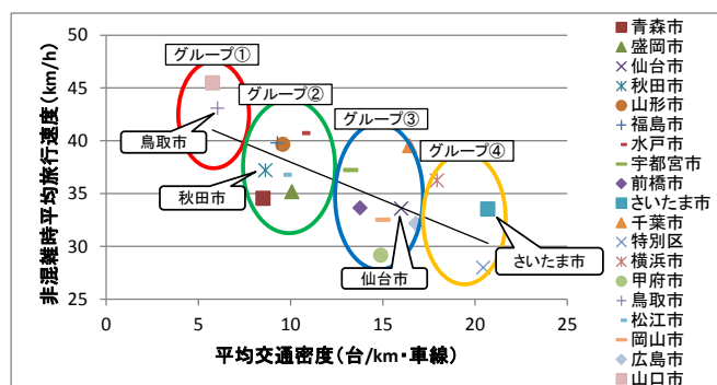
図-4 非混雑時平均旅行速度と平均交通密度との関係
