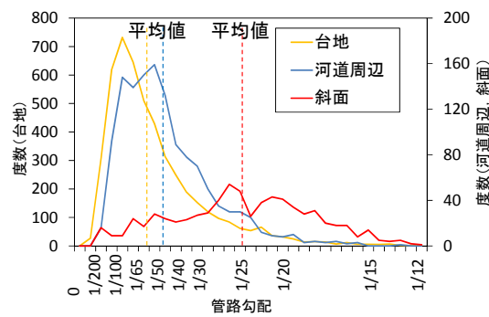
図-7 管路勾配の度数分布図
