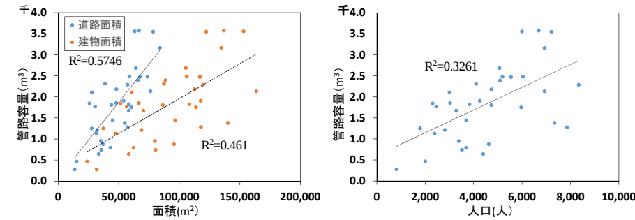
図-4 管路容量と道路・建物面積の関係 図-5 管路容量と人口の関係
