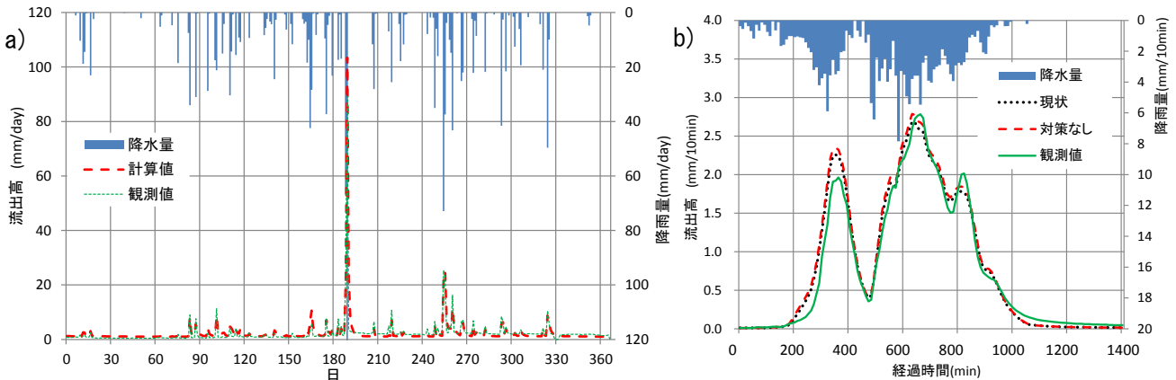
図-3 解析結果, a) 日単位の高ドログラフ, b) 10 分単位の高ドログラフの一例
