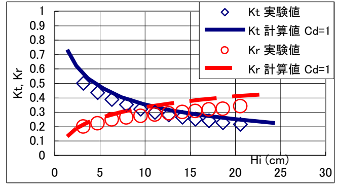
図3 ヘチマロン ( d=60\text{cm} T=3\text{s} )
