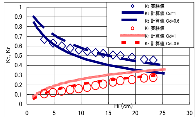
図5 ヘチマロン+円柱群 ( d=60\text{cm} T=3\text{s} )
