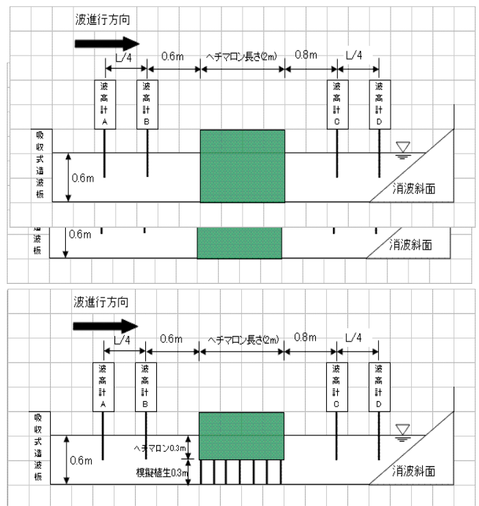
図 1 実験装置
