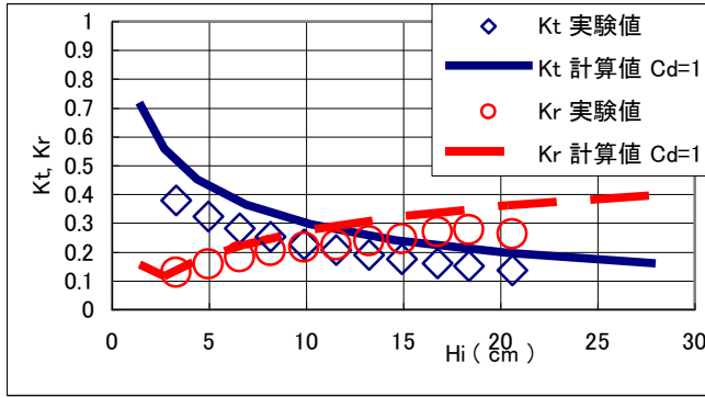
図2 ヘチマロン ( d=60\text{cm} T=2\text{s} )
