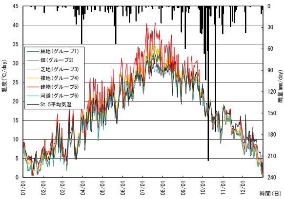
図-4 土地利用グループ毎の日平均地表面温度 (St. 5 の気温を与えた領域：case 0)
