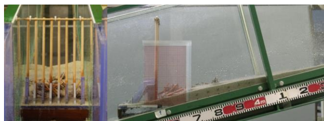
(c) Q=0.33 \text{ l/s} 流木混じり
