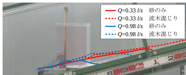
写真-4 土砂の捕捉形状の比較
