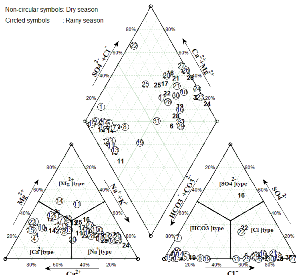
図-4 パイパーダイアグラム適用結果
