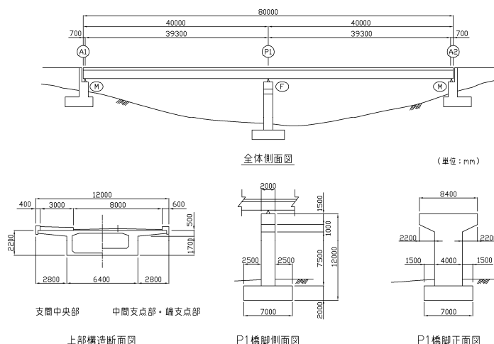
図1 解析対象橋梁
