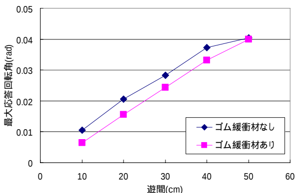
図3 橋脚基部の最大応答回転角と桁遊間の大きさの関係
