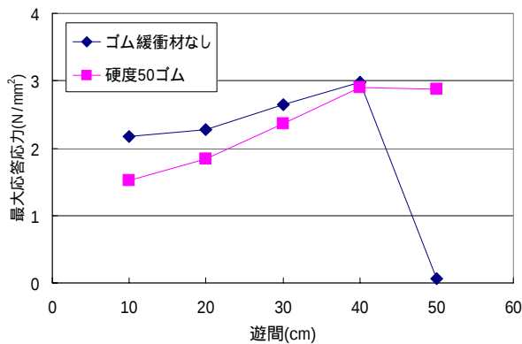
図2 橋桁端部の最大応答応力と桁遊間の関係
