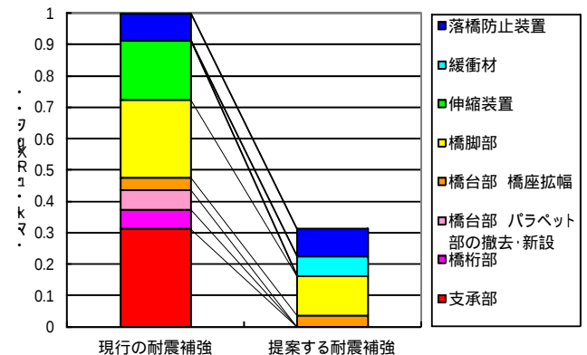
図4 提案する耐震補強のコスト削減効果
