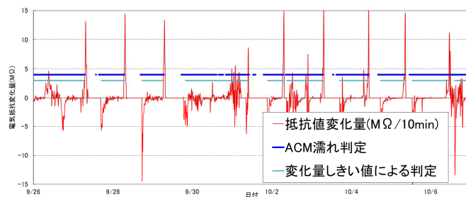
図-4 電気抵抗の変化量と ACM センサとの比較
