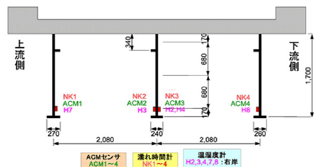
図-2 計測器取り付け位置(右岸側断面)
