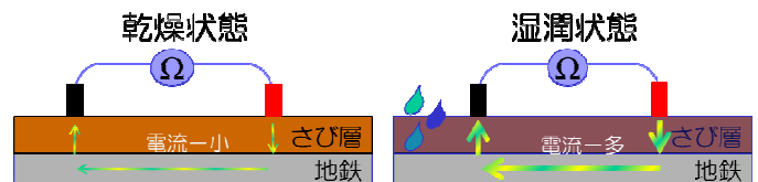
図-1 濡れの測定概念
