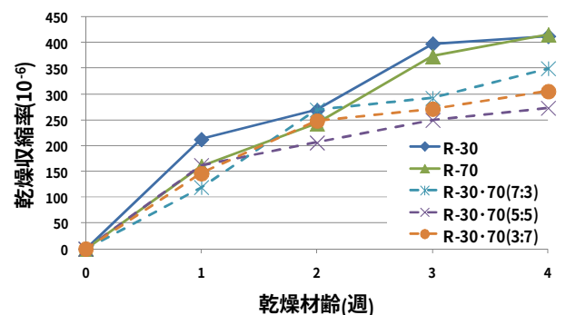
図-4 各配合の試験材齢における乾燥収縮率
