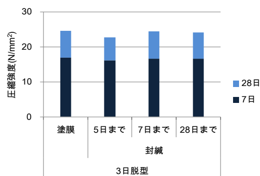
図-3 3 日脱型の塗膜養生と封緘養生の圧縮強度
