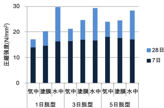
図-2 各養生条件の圧縮強度
