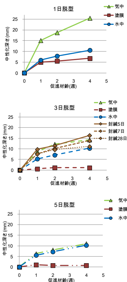
図-4 各養生条件の中性化深さ
