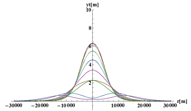
図-4 海底面の変位終了時の海面の変位 T=0, 1, 5, 10, 20, 30, 40, 50, 60, 80, 100 [s] の比較
