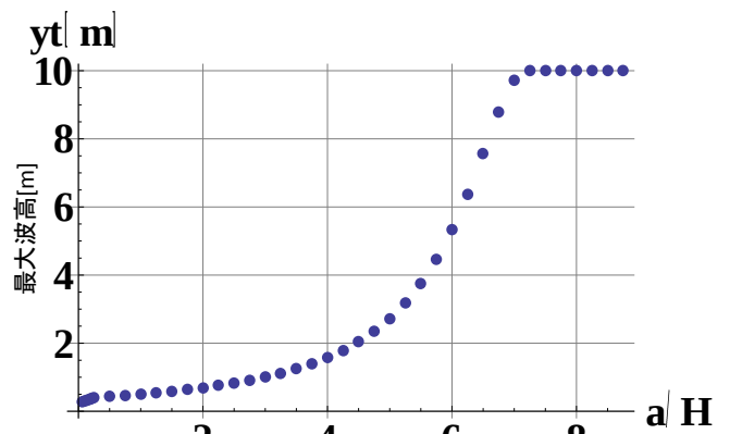
図-6 変位を起こす円区域の半径 a[m] と 水面の変位の最高点との関係
