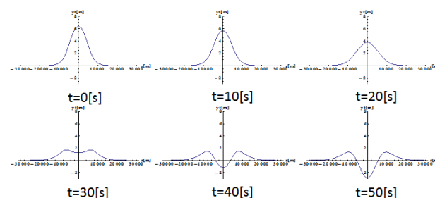
図-3 計算例, 海面の時系列変化 D=10 [m], H=4000 [m], a=5000 [m], T=0 [s] の場合
