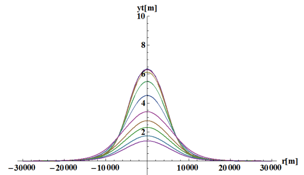
図-5 最大波高時の海面の変位 T=0, 1, 5, 10, 20, 30, 40, 50, 60, 80, 100 [s] の比較
