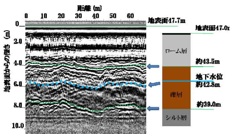
図-2 ボーリングデータとレーダプロファイル（赤実線）
