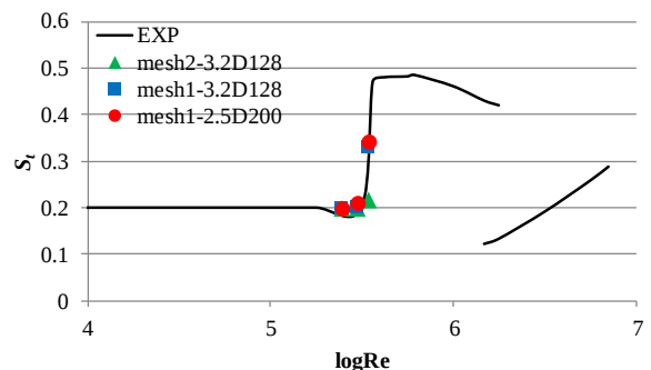
図-2 Strouhal 数 S_L の実験結果 2) と解析結果の比較
