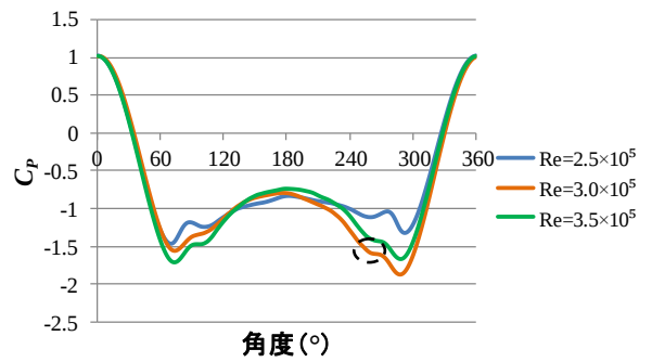
図-3 円柱まわりの平均圧力係数 C_p (mesh2-2.5D200)
