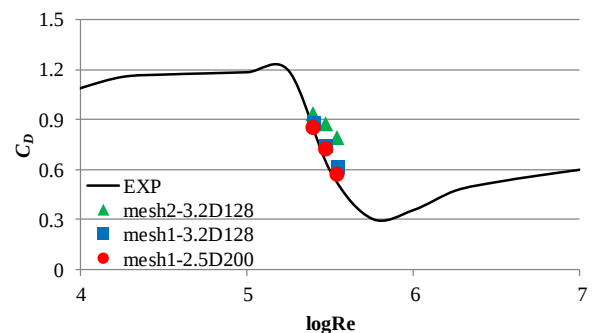
図-1 抗力係数 C_D の実験結果 1) と解析結果の比較
