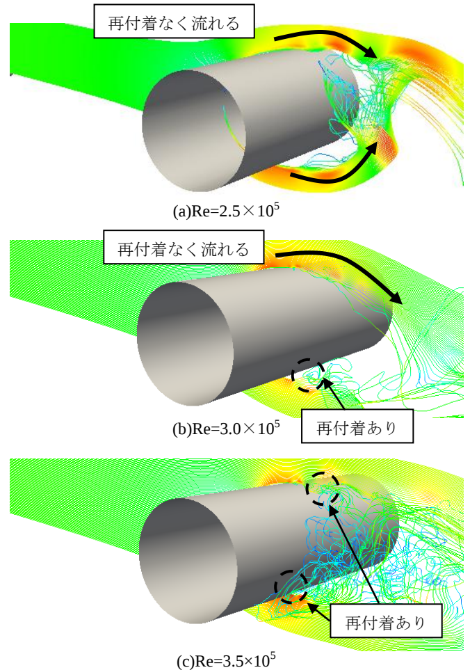
図-4 臨界 Re 数付近の流線図(mesh1-2.5D200)
