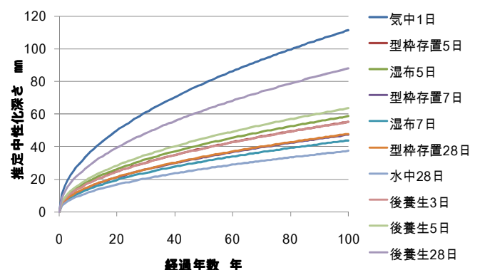
図-5 BB を用いた場合の劣化予測
