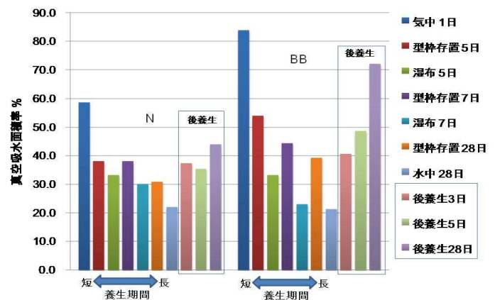
図-1 養生条件による真空吸水面積率
