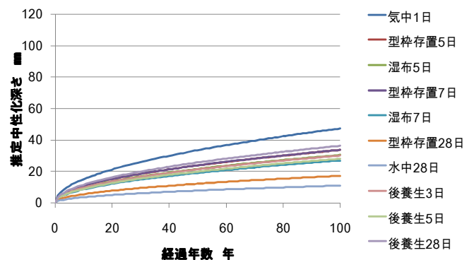
図-4 N を用いた場合の劣化予測
