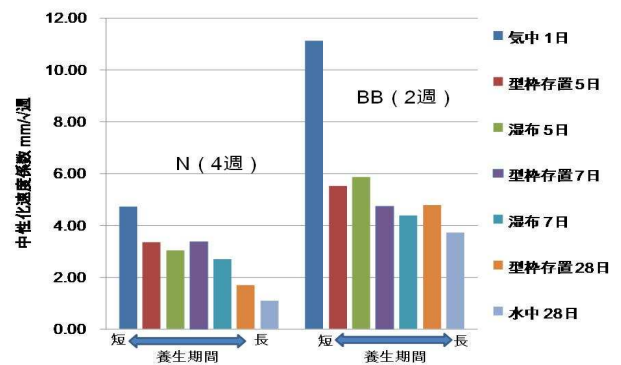
図-2 養生条件による中性化速度係数
