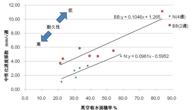
図-3 真空吸水面積率と中性化速度係数の関係
