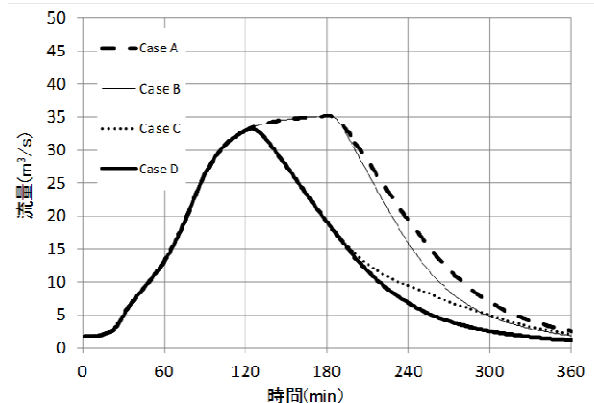
図-9 雨水貯留タンクからの放流シミュレーションによる方南橋地点の河道流量
