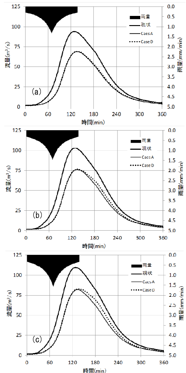
図-6 中央集中型降雨による方南橋地点の計算河道流量，(a) 10 年確率，(b) 15 年確率，(c) 20 年確率
