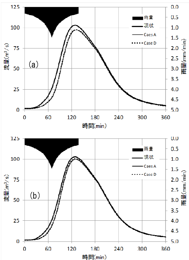
図-7 豪雨直前の初期貯留量を考慮した場合の方南橋地点の河道流量，(a)下位 25%値，(b)下位 50%値
