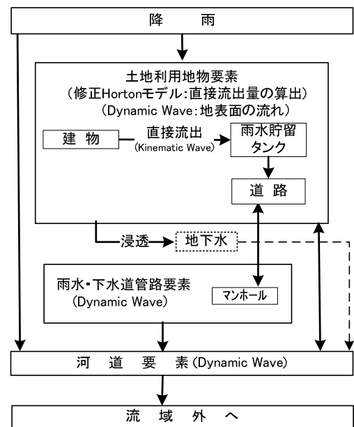
図-5 TSR モデルの概要
