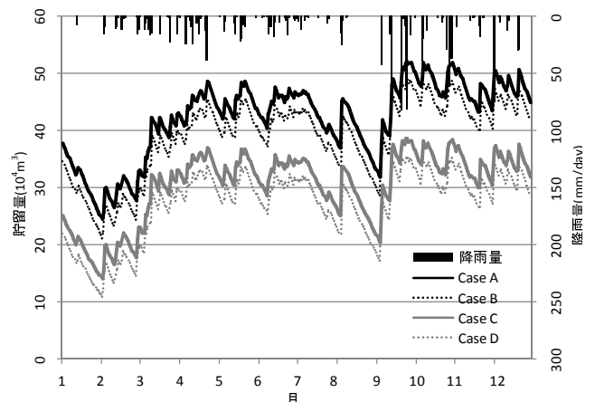
図-4 総雨水貯留量の時系列変化の一例
