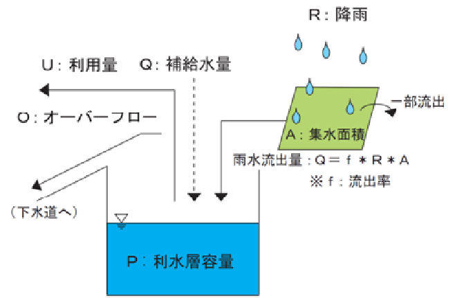
図-2 雨水貯留タンクモデル図
