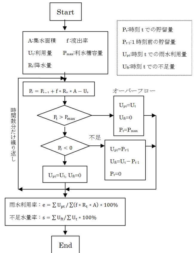
図-3 雨水貯留タンクフロー
