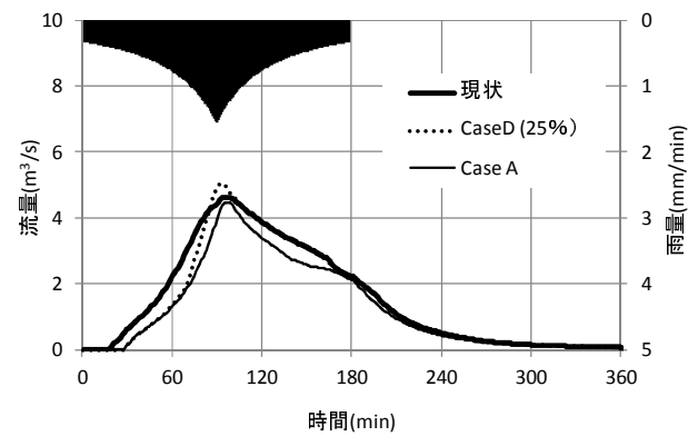
図-8 小排水区から河道への排水量
