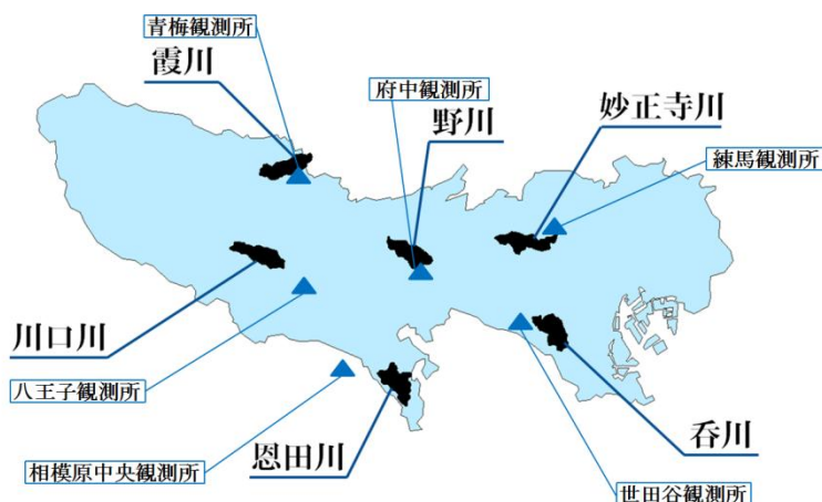
図-2 対象流域
