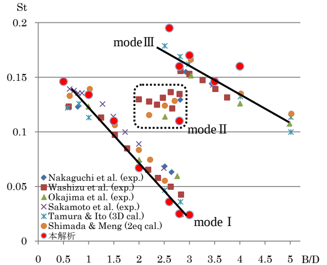
図-2 辺長比毎のストローハル数(既往の結果との比較)
