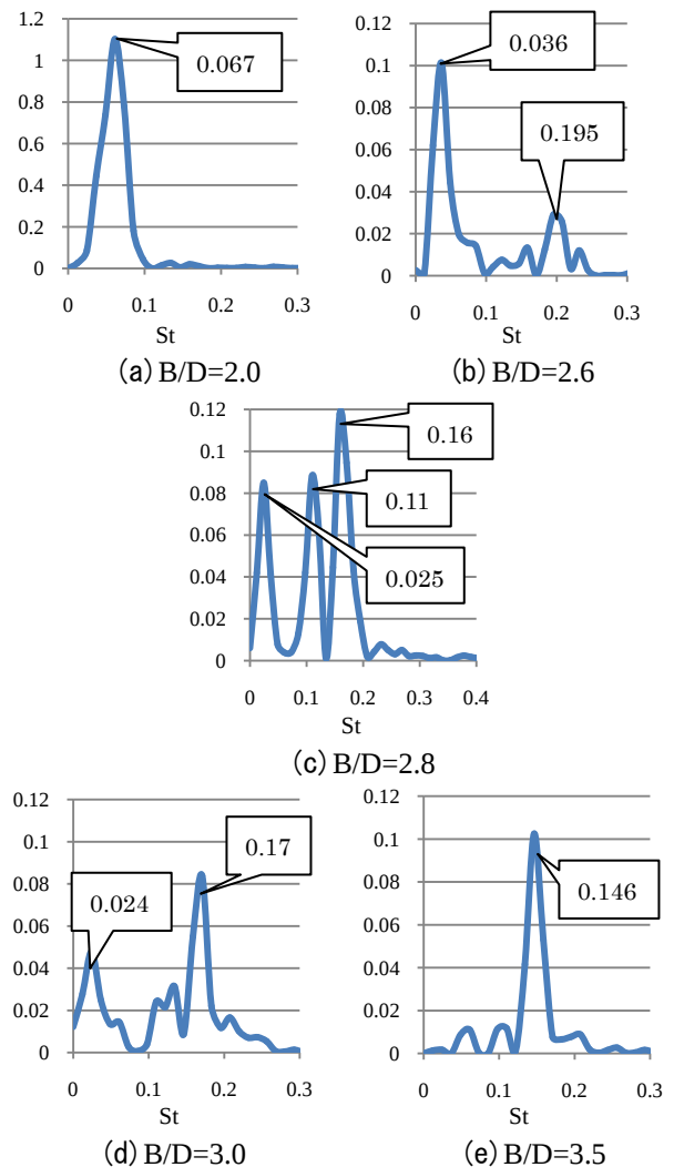
図-3 揚力のスペクトル
