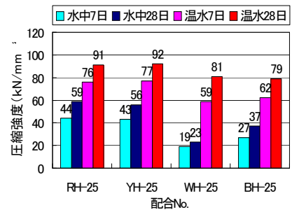
図 3 圧縮強度試験結果 (W/P 25%)
