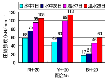
図 2 圧縮強度試験結果 (W/P 20%)
