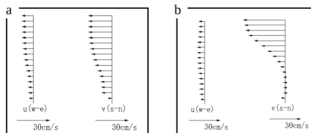
図4:St.4の流速の鉛直分布(a:ケース1, b:ケース2)
