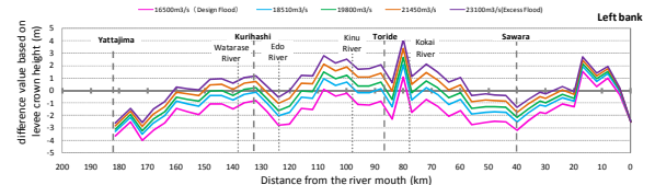
図－5 左岸側の天端高を基準とした際の水位との差分値
