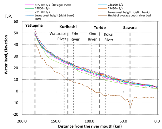
図－3 計画高水流量時と仮定した超過洪水時の水位と天端高の比較
