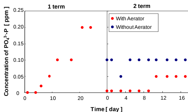
図.4 水質環境および酸素供給の相異による液中 \text{PO}_4^{3-} -P 濃度変化
