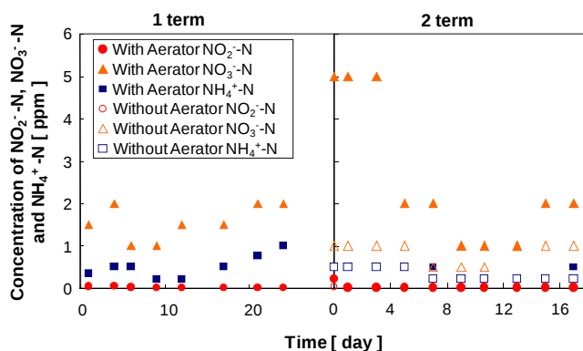
図.3 水質環境および酸素供給の相異による液中 T-N 濃度変化
