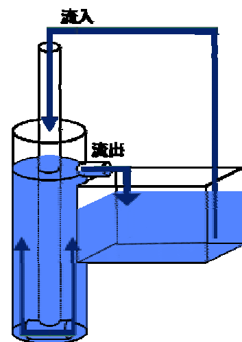
図-2 流動床反応槽構造
