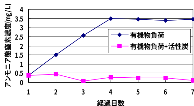
図-1 アンモニア態窒素濃度の推移
