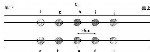
図-2 鉄筋近傍熱電対設置位置
