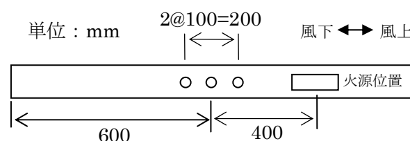
図-3 シース熱電対設置位置
