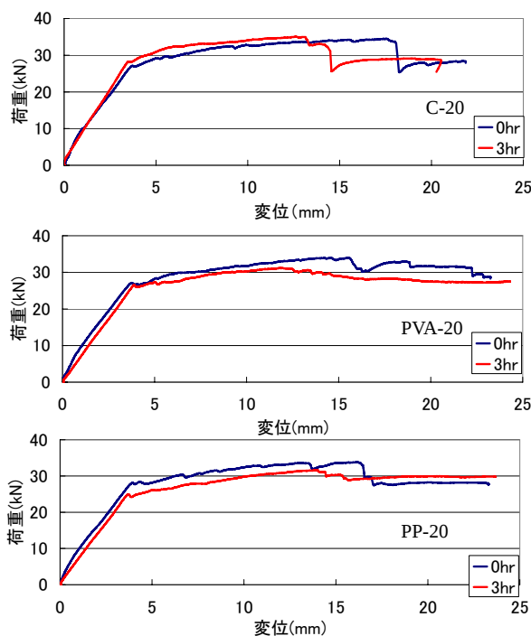
図-7 荷重-変位曲線
