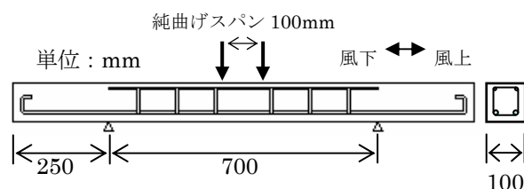
図-1 鉄筋配筋図
