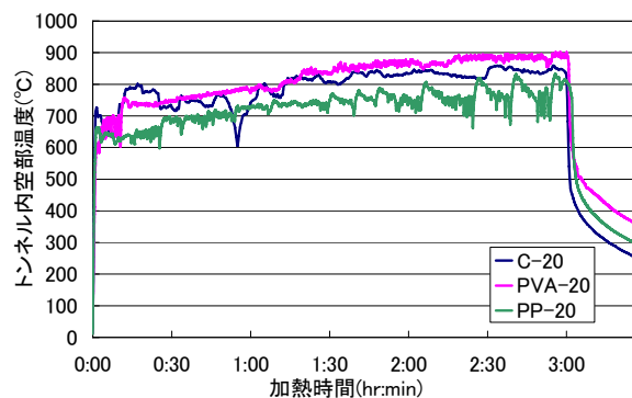
図-4 温度-時間曲線
