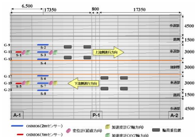
図-4 計測器設置情况
