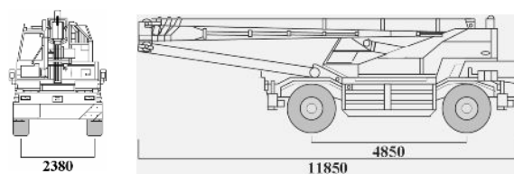
図-3 検測車輛図
