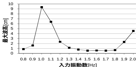
図-2 入力振動数における最大波高
