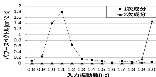
図-4 入力振動数におけるパワースペクトル
