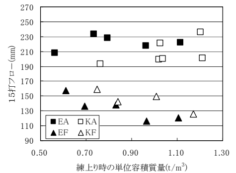
図-4 単位容積質量とフローの関係
