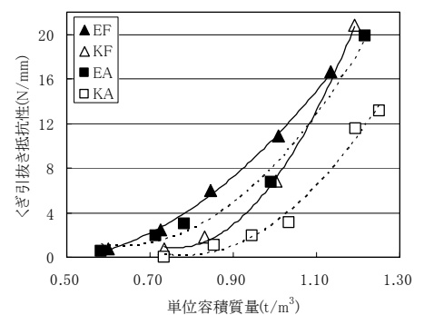
図-6 単位容積質量とくぎ引抜き抵抗性の関係
