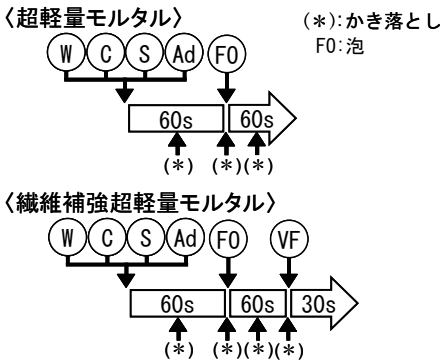
図－１ モルタルの練混ぜ方法
