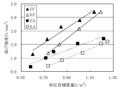
図-5 単位容積質量と曲げ強度の関係
