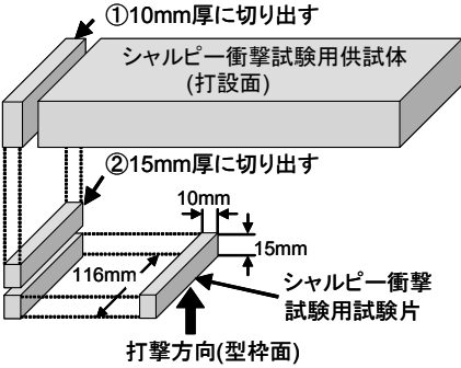
図－３ シャルピー衝撃試験用試験片の作製方法
