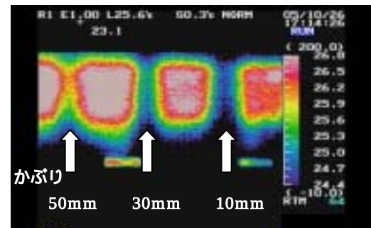
(b) 鉄筋を配置した供試体のうら面にお ける温度分布図
