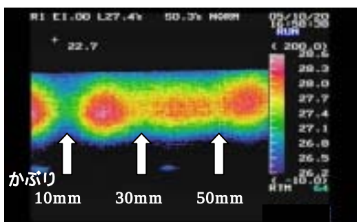
(a) 鉄筋を配置した供試体のおもて面にお ける温度分布図
