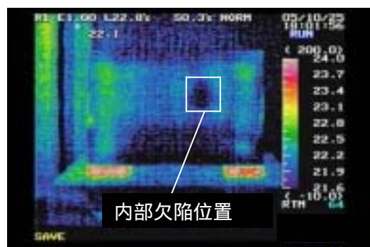
(b) マイクロ波を照射した面とは逆側の面（うら面） の温度分布図
