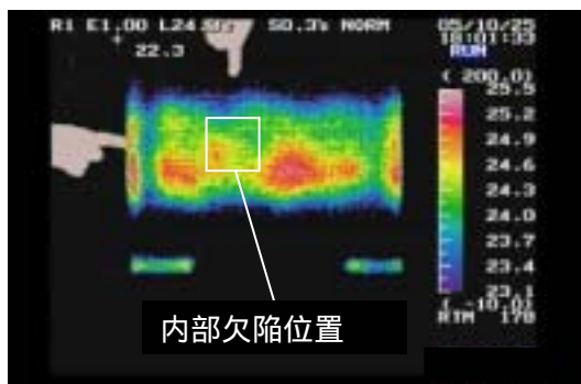
(a) マイクロ波を照射した面（おもて面） の温度分布図
