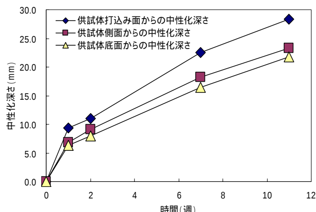
図-5 中性化深さと中性化促進期間との関係 (W/C=65%)
