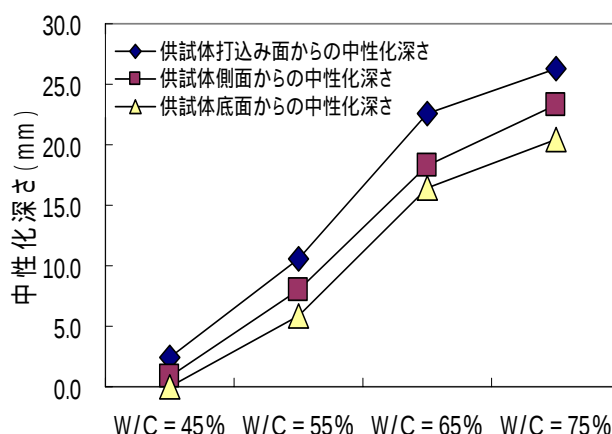
図-3 打込み面・側面・底面における中性化深さ
