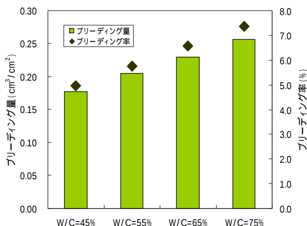
図-2 ブリーディング試験
