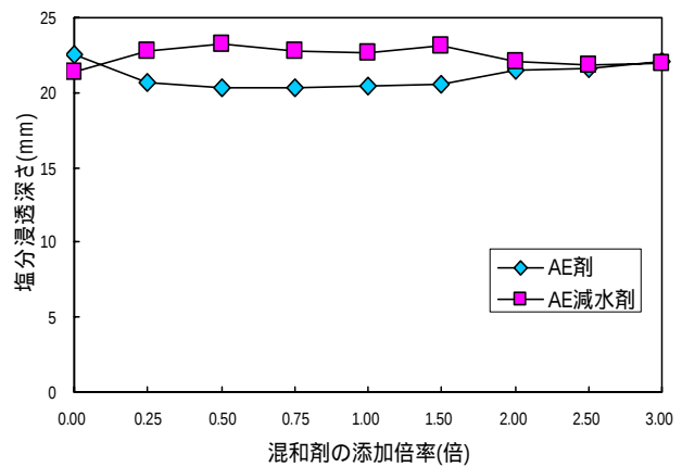
図 - 2 添加率変化による塩分浸透深さ
