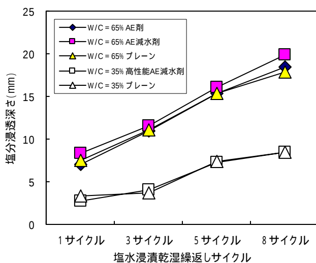
図 - 3 塩水浸漬乾湿繰返し試験結果
