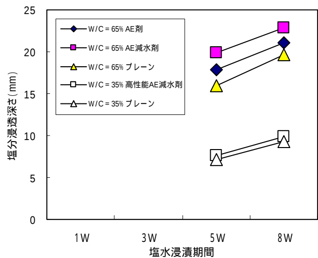
図 - 4 塩水全漬試験結果
