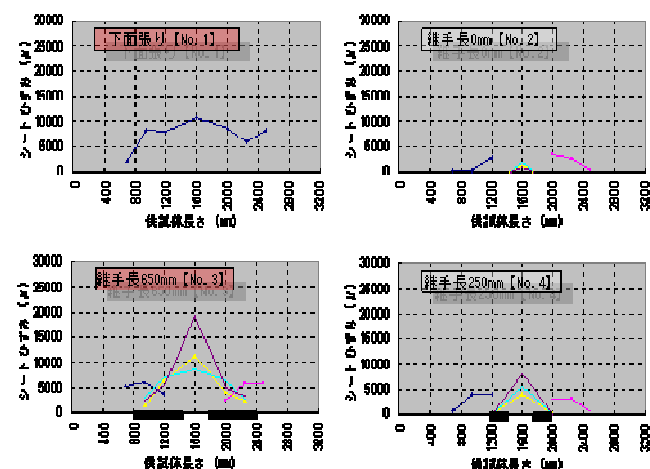
図 5 繊維シートの軸方向ひずみ分布性状
