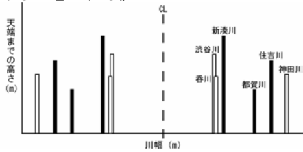
図－1 河川横断面図の比較
