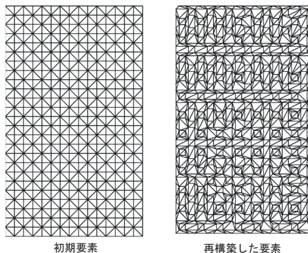
図-3 解析要素
