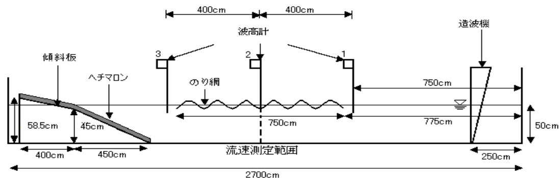
図-1 実験水路概要図
