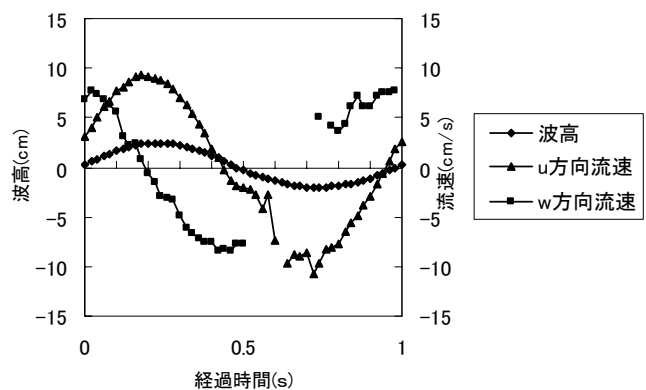
図-7 波高・流速（のり付網、深さ 12\text{cm} ）
