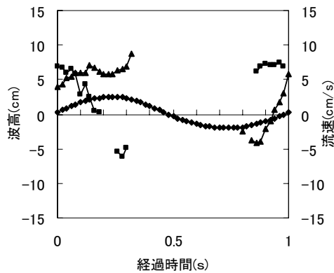
図-6 波高・流速（のり付網、深さ 10\text{cm} ）
