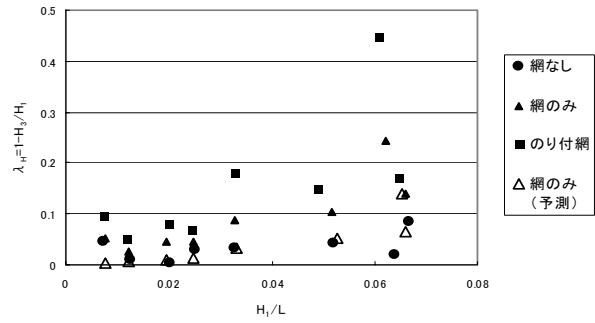
図-3 波形勾配と波高減衰率との関係
