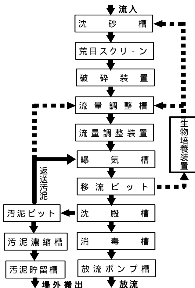
図 - 1 浄化槽のフロ - シ - ト
