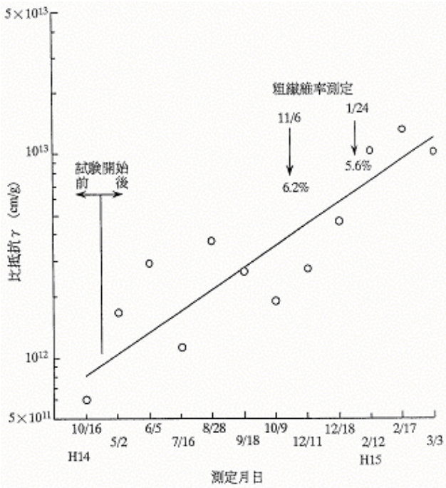
図 - 2 曝気槽活性汚泥の比抵抗の変化
