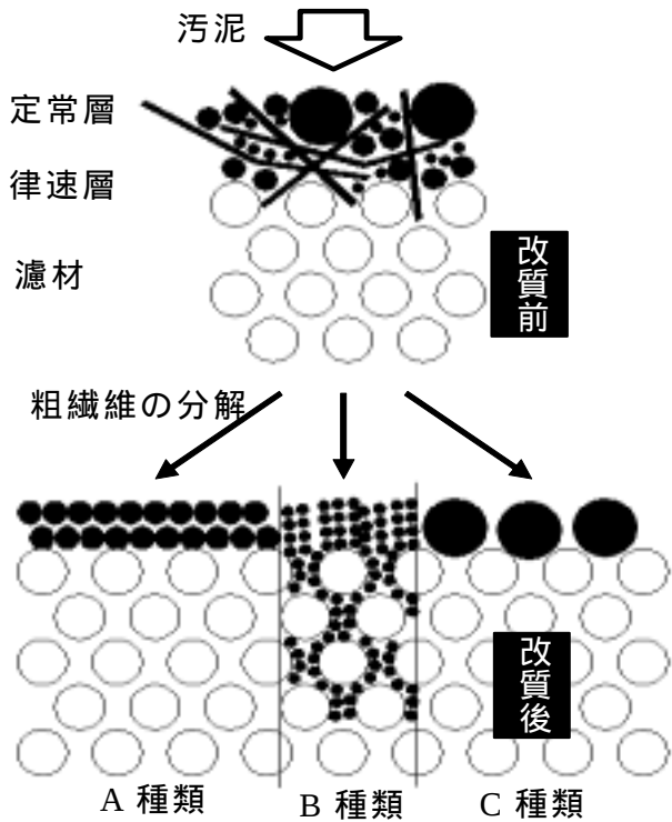
図 - 3 汚泥の脱水モデル形態
