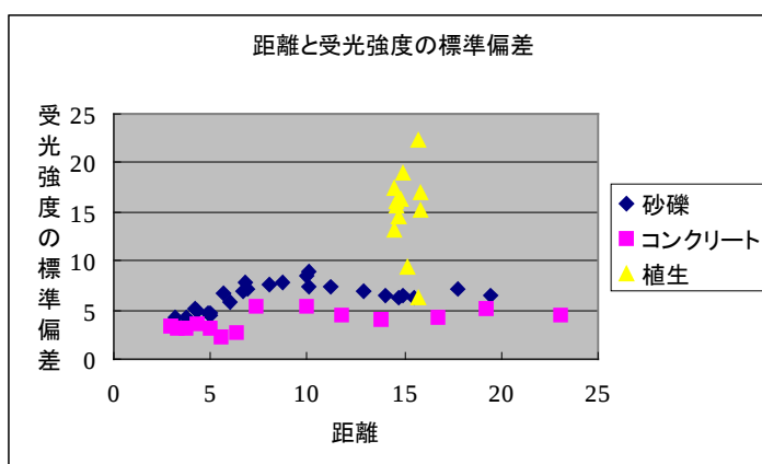
図-3 河道内対象物の距離と受光強度の標準偏差の関係
