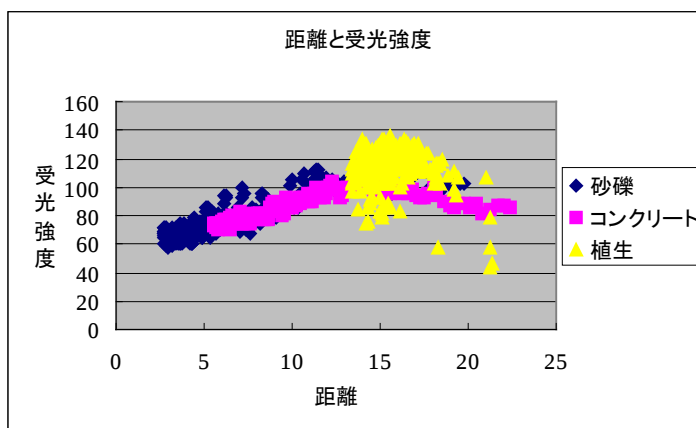
図-2 河道内対象物の距離と受光強度の関係
