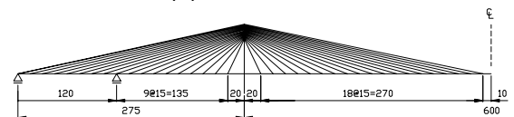
(b) 600m モデル
