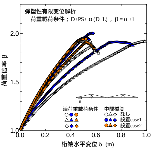
図-5 600m モデルの桁端荷重-変位曲線
