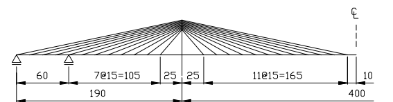
(a) 400m モデル
