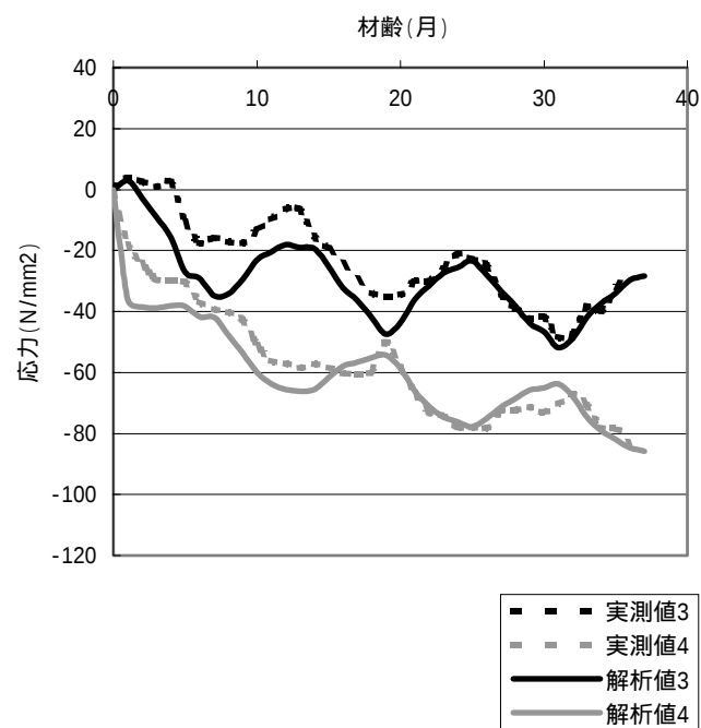
図-3 柱上部の鉄筋応力の経時変化
