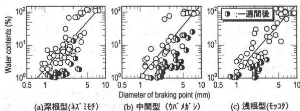
図-6 水分量と直径の関係
