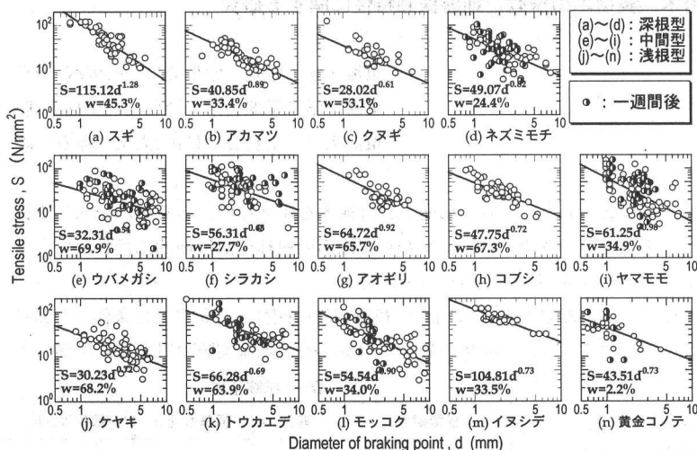
図-3 根系の引張強度 S と直径 d
