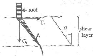
図-1 根系のせん断抵抗力 21)
