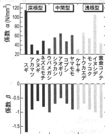
図-4 係数 \alpha と \beta の比較
