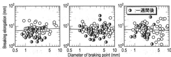
図-5 根の伸長量(破断時)と直径の関係
