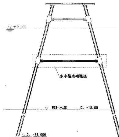
図-1 橋脚構造図
