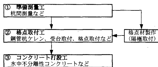
図-5 施工フロー図
