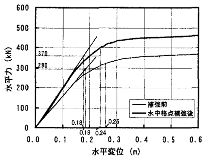
図-2 水平力-変位履歴図
