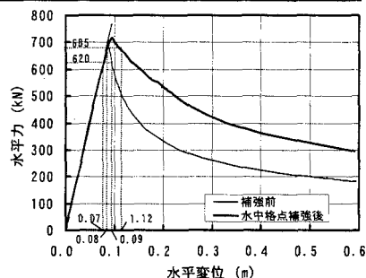
図-4 座屈先行型の水平力-変位履歴図
