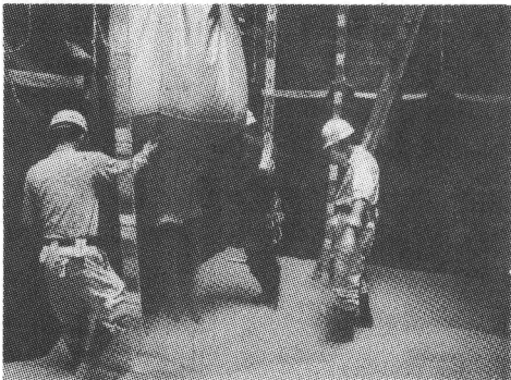
写真-1 トシバックによる砂の投入状況(例)
