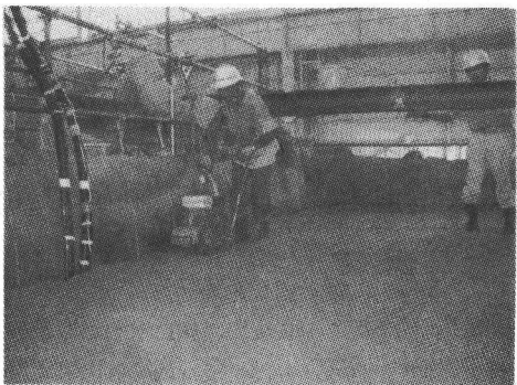
写真-2 プレートコンパクタによる締め固め状況(例)
